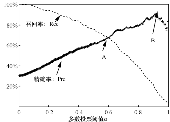
图 7 WRF 分类器对空巢用户识别泛化性能曲线
