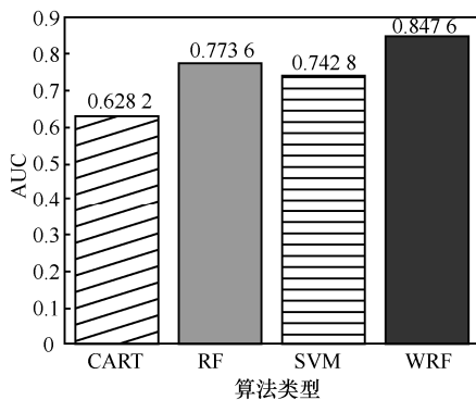
图 6 不同算法下空巢用户识别 AUC 值
